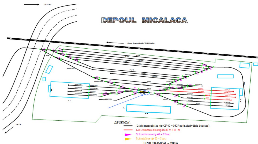
Planul general al depoului Micălaca
