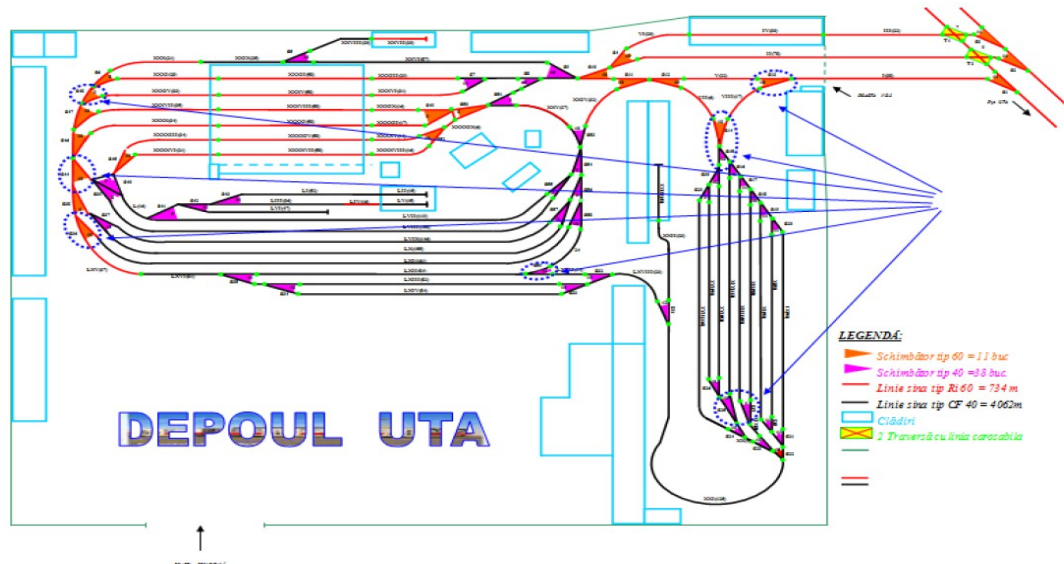
Planul general al depoului UTA
